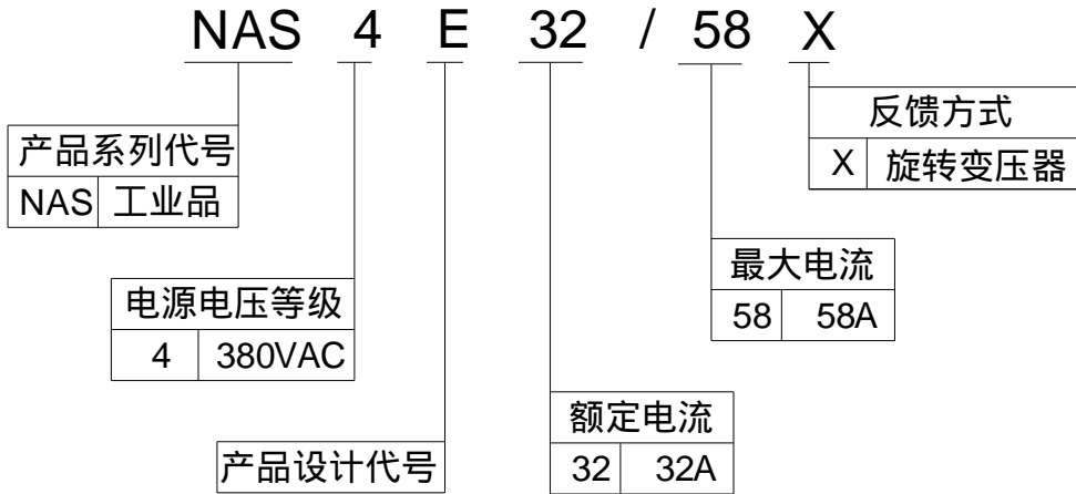
图 2-1 驱动器命名规则
